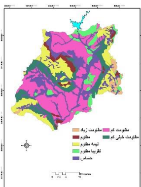
شکل ۱۱. نقشه مقاومت لتولوژیک
