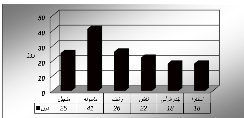
شکل ۲: مجموع فراوانی وقوع سالانه فون در ایستگاههای مورد مطالعه (۲۰۰۶-۲۰۱۵)
