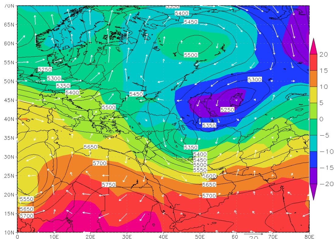
شکل ۱۱: نقشه ترکیبی ارتفاع ژ.پ تراز ۵۰۰ ه.پ (کنطور)، دما (°C) (پهنه رنگی) و بردارهای سمت و سرعت باد (m/s) تراز
