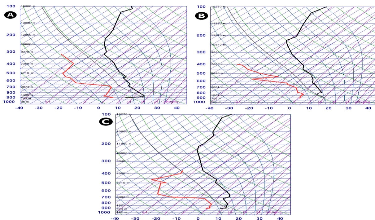
شکل ۶) نمودارهای اسکیتی-logP (لگاریتمی فشار) برای ایستگاه رادیوسوند مشهد برای الگوی پرفشارمهاجر در ساعت ۰۰۰ گرینویچ. در تمامی نمودارها، خط های ضخیم سیاه و قرمز به ترتیب معرف دمای هوا و دمای نقطه شبنم می باشند. ( http://weather.uwyo.edu )
