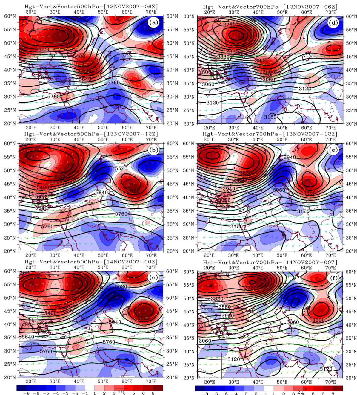
شکل ۳) وضعیت همدیدی در الگوی پرفشار مهاجر برای ساعات مختلف روزهای آلوده. ارتفاع ژئوپتانسیل (کنتورها با حداصل ۲۵ ژئوپتانسیل متر)، تلاوایی نسبی (رنگ ها 10^{-5} s^{-1} ) و باد برداری (پیکان های سبز رنگ) در تراز ۵۰۰ (سمت چپ) و تراز ۷۰۰ هکتوپاسکال (سمت راست).
