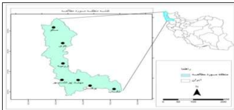
شکل ۱: موقعیت ایستگاه‌های هواشناسی محدوده‌ی مطالعه در استان آذربایجان غربی.
