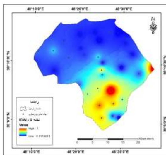
شکل ۳: نقشه‌ی فازی به روش IDW برای سال آبی ۱۳۶۰.
