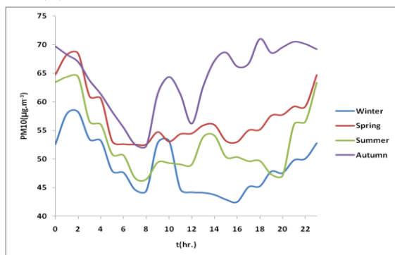
شکل ۸. چرخه‌ی شبانه‌روزی میانگین ساعتی، الف) تندى باد، ب) جهت باد، پ) دما، ت) CO و ث) PM ۱۰ در فصل‌های مختلف سال ۲۰۰۷.
