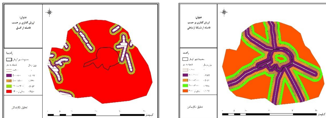
شکل (۳). ارزش گذاری برحسب فاصله از شبکه ارتباطی
