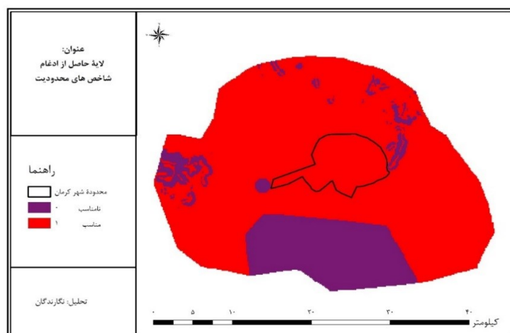
شکل (۶): لایه حاصل از ادغام شاخص های محدودیت
