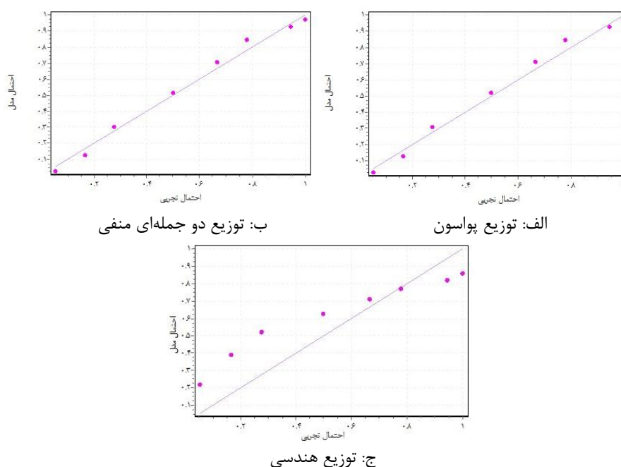
شکل (۲). نمودار احتمال - احتمال (p-p) برای مشاهدات جدول ۴ ایستگاه بانه (۱۹۹۲-۲۰۱۴)
