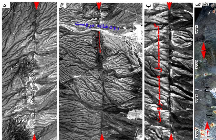
شکل (۱۰) تاثیر نوزمینساخت گسل مروت در ایجاد شواهد ژئومورفیک؛ (الف) تصویر ASTER اثر گسل دهشیر را نشان می‌دهد، موقعیت تصاویر ب، ج، و د بر روی آن مشخص شده است. (ب) دره‌های خطی منطبق بر اثر گسل مروت بر روی مخروط افکنه مروت، (ج) رودخانه‌های جایجا شده، رودخانه‌های بی‌سر، پشته‌های مسدود کننده در امتداد گسل مروت، (د) جابجاشدگی‌های افقی و انحراف مسیل‌ها
