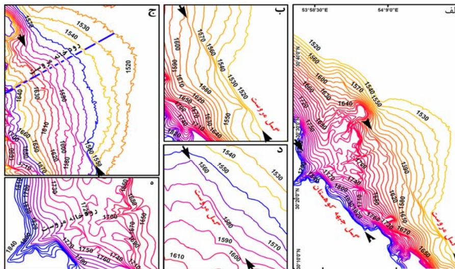
شکل (۹) آشکارسازی تاثیر نوزمینساخت به کمک الگوی منحنی‌های تراز در مخروط افکنه مروت
