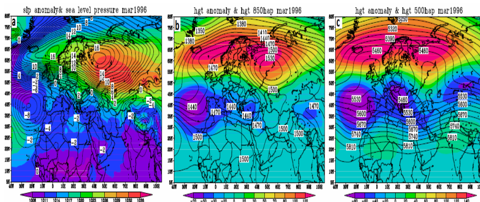
شکل (۹) میانگین و ناهنجاری فشار تراز دریا (a) و ارتفاع ژئوپتانسیل تراز ۸۵۰ و ۵۰۰ هکتوپاسکال (c) در مارس ۱۹۹۶
