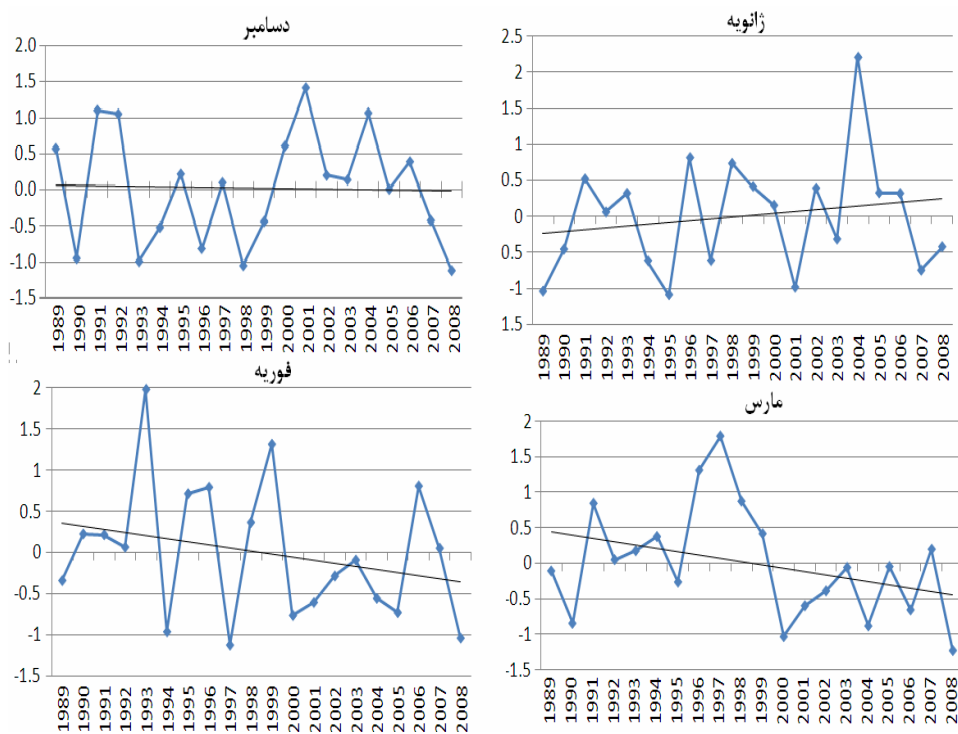
شکل (۲) روند تغییرات شاخص Z در جنوب غرب ایران
