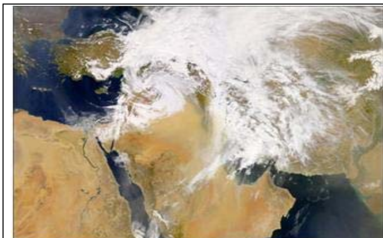
شکل (۱۲) : تصویر ماهواره ای سامانه گرد و غباری ۲۶ مارس ۲۰۰۳.
