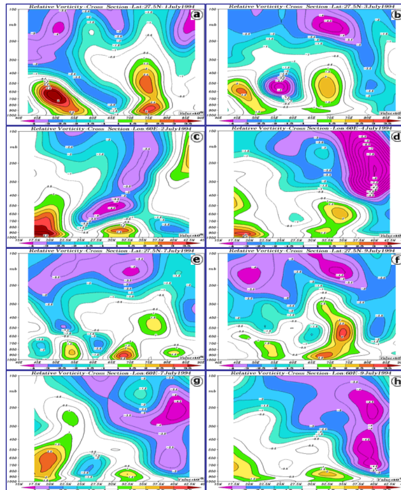
شکل ۷. نیمرخ قائم تاوایی نسبی با استفاده از داده‌های ۱۲ تراز فشاری، برحسب s^{-1} \times 10^{-5} برای روزهای دهه اول جولای ۱۹۹۴. (a, b, e, f) نیمرخ قائم در امتداد عرض ۲۷٫۵ درجه شمالی و (c, d, g, h) نیمرخ قائم در امتداد طول ۶۰ درجه شرقی. در شکل‌ها از نشان‌دادن مقادیر تاوایی بین -0.5 \times 10^{-5} s^{-1} و 0.5 \times 10^{-5} s^{-1} صرف‌نظر شده است.
