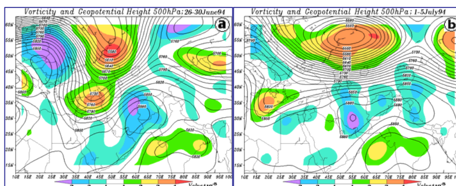
شکل ۵. نقشه‌های ترکیبی متوسط پنج روزه تراز 500 هکتوپاسکال. (a) دوره پنج روزه قبل از شروع بارش (۲۶ الی ۳۰ ژوئن ۱۹۹۴). (b) دوره پنج روزه دارای بارش فراگیر (۱ الی ۵ جولای ۱۹۹۴). در نقشه‌ها تاوایی نسبی برحسب 10^{-5} s^{-1} و ارتفاع ژئوپتانسیل برحسب متر می‌باشد. در شکل‌ها از نشان تاوایی -1 الی +1 ( 10^{-5} s^{-1} ) صرف‌نظر گردیده است.
