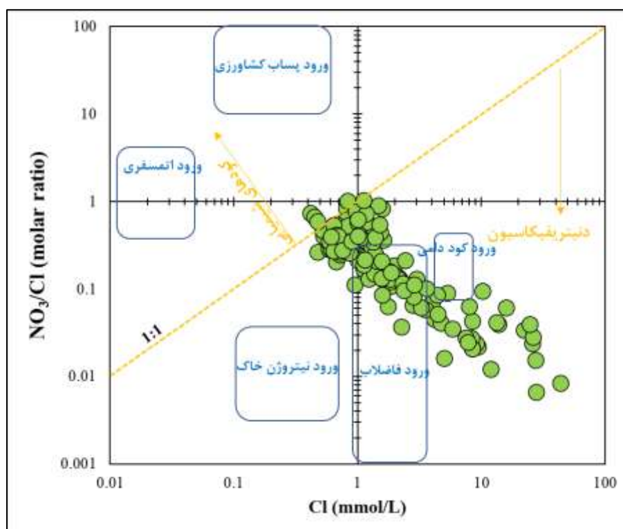
شکل (۱۲). شناسایی منابع احتمالی نیترات در آب زیرزمینی بر اساس نسبت \text{NO}_3/\text{Cl} در مقابل \text{Cl}
