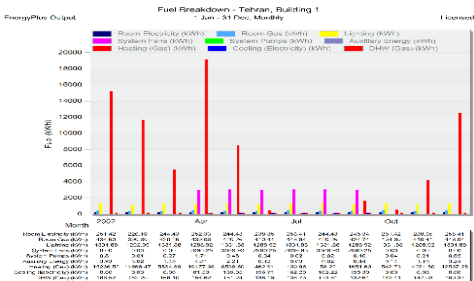
شکل (۶). نتایج مصارف مختلف برق و گاز بر حسب کیلووات ساعت در ماه‌های مختلف
