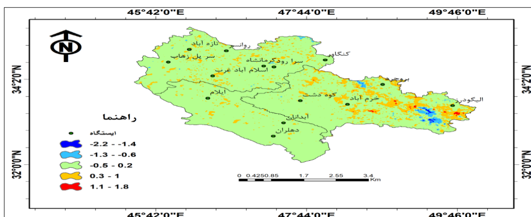
شکل (۹). روند تغییرات روزهای برف‌پوشان فصل بهار
