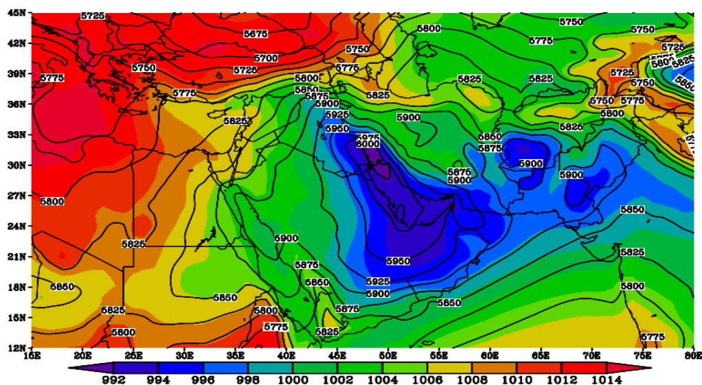
شکل (۶). نقشه ترکیبی فشار سطح زمین (نقشه رنگی) و وضعیت ضخامت جو (کنتورهای سیاه و سفید) در ساعت ۱۵/۳۰ روز ۱۳ ژوئیه ۱۹۸۸
