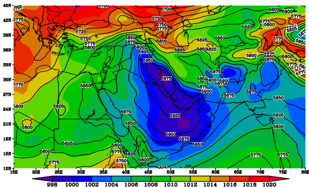
شکل (۱۴). نقشه ترکیبی فشار سطح زمین (نقشه رنگی) و وضعیت ضخامت جو (کنتورهای سیاه و سفید) در ساعت ۱۵/۳۰ روز ۳ اوت ۲۰۰۱
