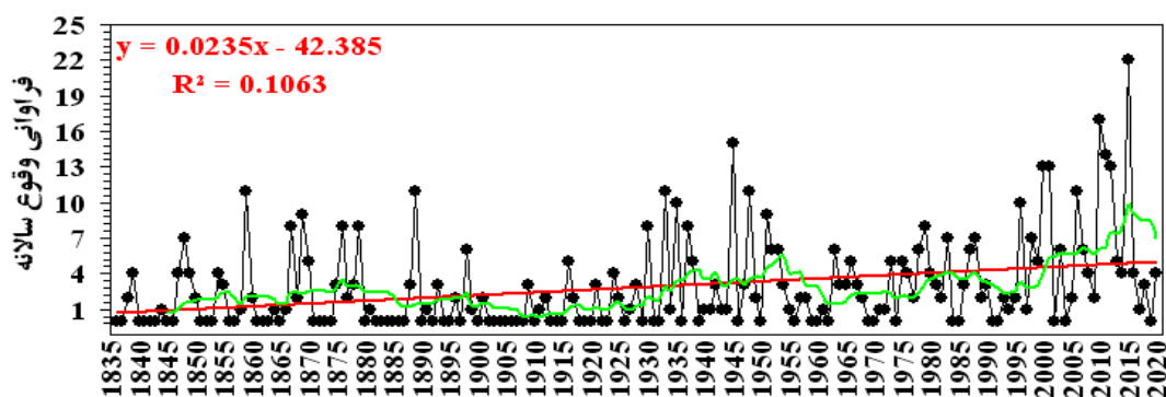
شکل (۲). فراوانی سالانه وقوع دمای بالای ۵۰ درجه سانتی‌گراد (۱۸۳۶ تا ۲۰۲۰). خط فسفری رنگ میانگین متحرک ۱۰ ساله و خط قرمز روند هستند.
