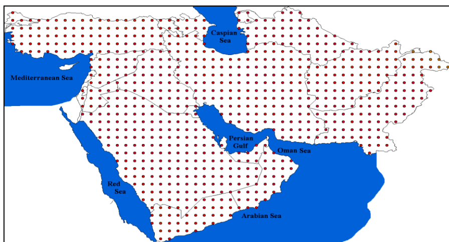
شکل (۱). نقشه منطقه مورد غرب آسیا با پوشش نقاط شبکه‌ای ۱×۱ درجه داده‌های واکاوی شده 20CR
