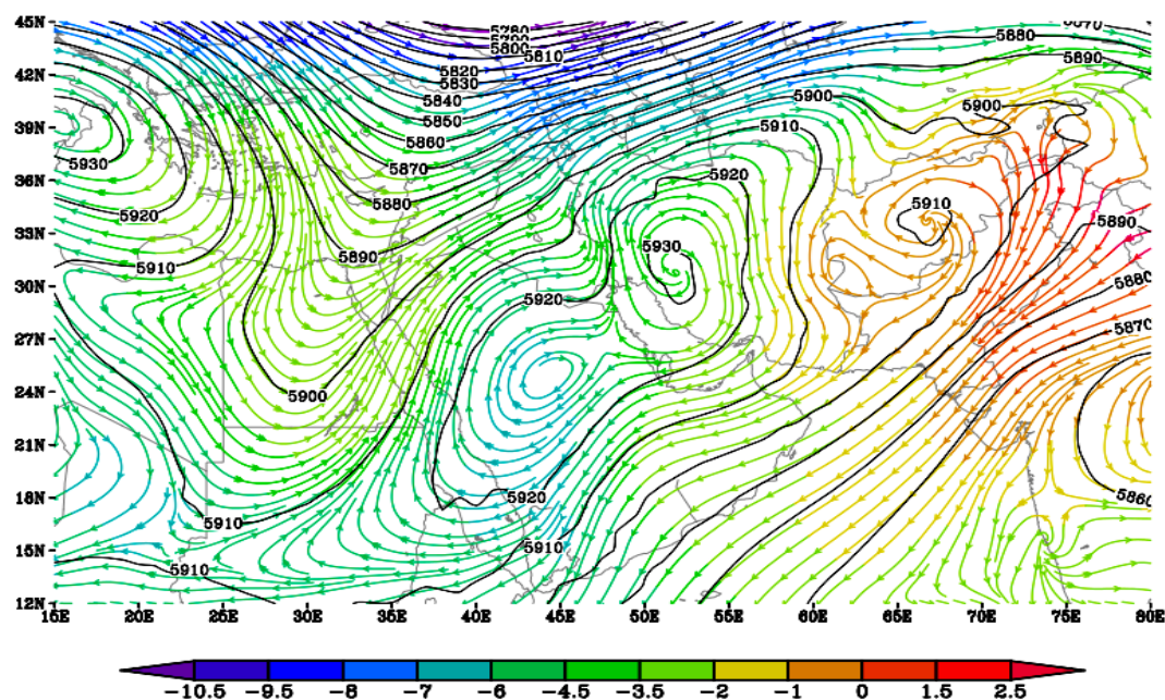
شکل (۱۹). نقشه ترکیبی وزش دمایی و ارتفاع ژئوپتانسیل تراز ۵۰۰ هکتوپاسکال در ساعت ۱۵/۳۰ روز ۱۵ ژوئیه ۲۰۱۵
