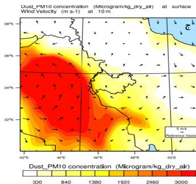
شکل (۷). پیش‌بینی توزیع غلظت گردوغبار توسط مدل WRF- chem (الف) نقشه ۱ / ۲۰۱۷/۱۱/ (ب) نقشه ۲ / ۲۰۱۷/۱۱/ (ج) نقشه ۳ / ۲۰۱۷/۱۱/
