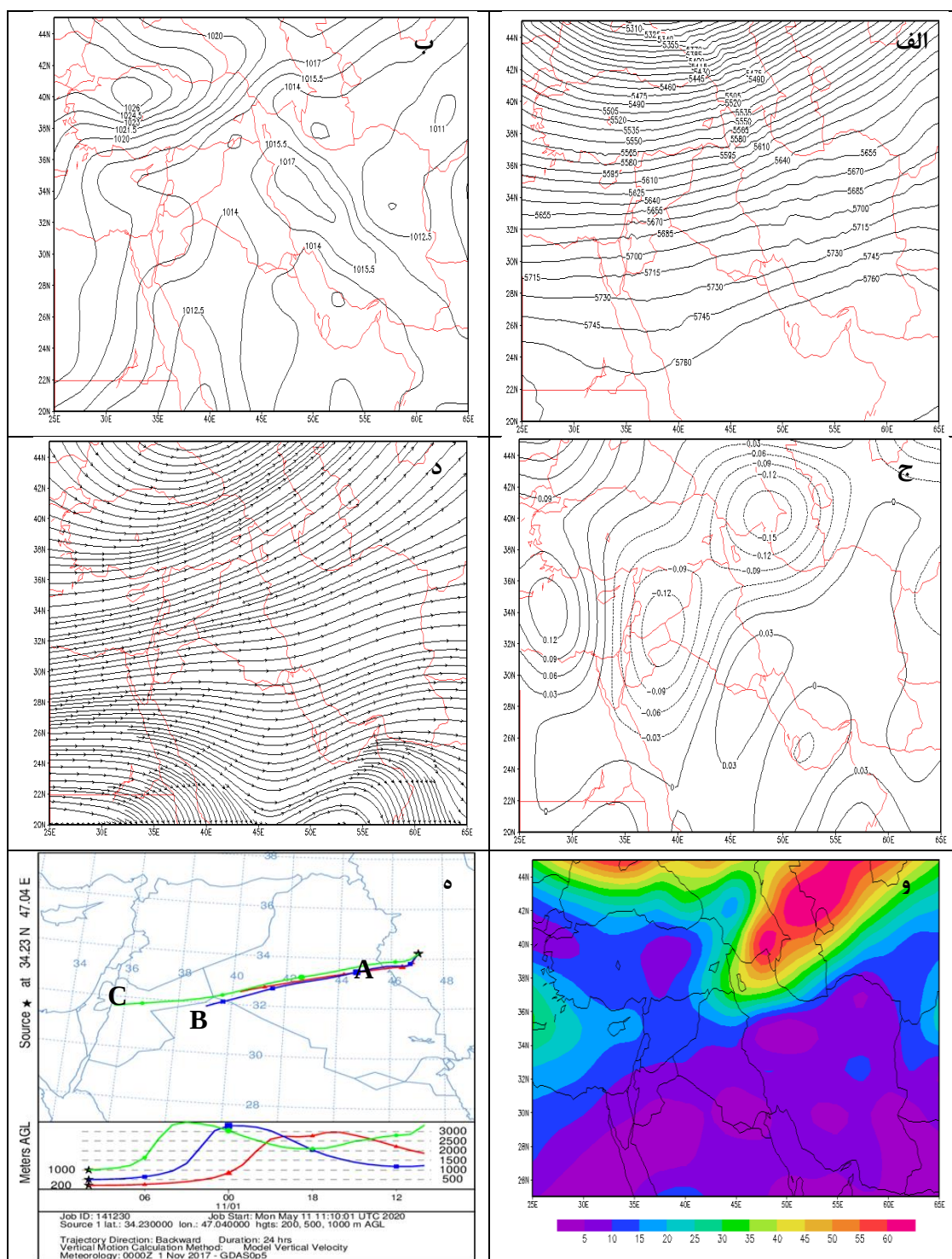
شکل (۲). الف) ارتفاع ژئوپتانسیل تراز ۵۰۰؛ ب) فشار سطح دریا؛ ج) امگای تراز ۷۰۰؛ د) جریان باد در تراز ۳۰۰؛ و) رطوبت ویژه ۷۰۰؛ ه) نقشه ردیابی ذرات گردوغبار HYSPLIT روز ۱ نوامبر ۲۰۱۷
