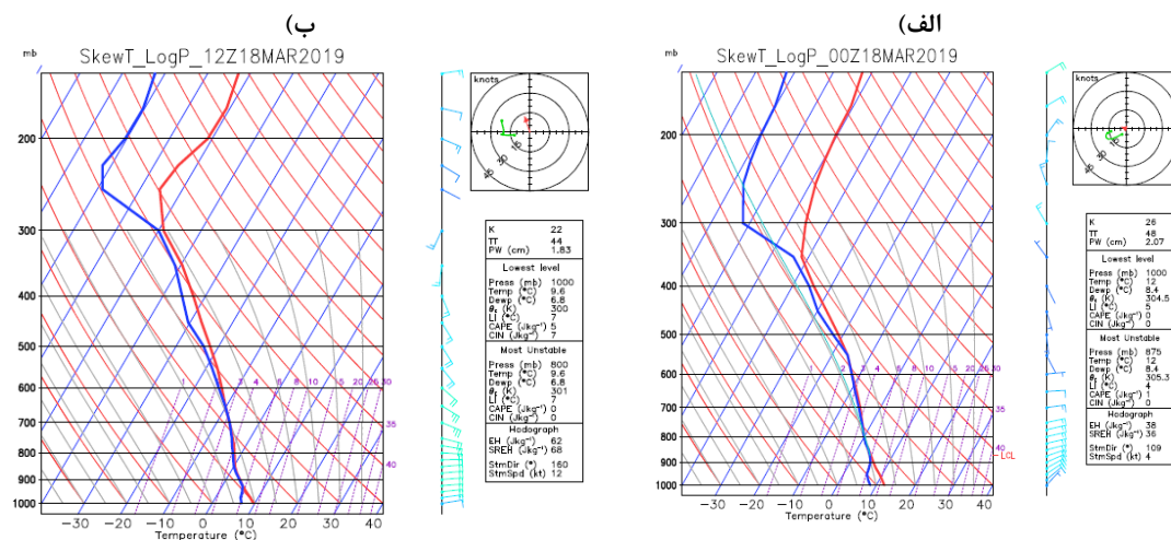
شکل (۸). الف) نمودارهای ترمودینامیکی ساعت ۰۰۰۰ و ب) ۱۲۰۰ گرینویچ روز ۲۷ اسفند ۱۳۹۷ ایستگاه گرگان
