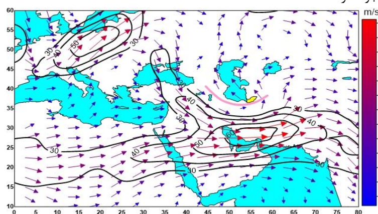
شکل (۹). میدان باد تراز ۳۰۰ هکتوپاسکال (متر بر ثانیه) در ساعت ۰۰۰۰ گرینویچ روز ۱۸ مارس ۲۰۱۹
