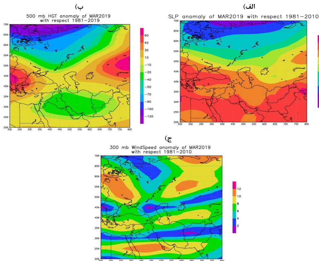
شکل (۶). ناهنجاری (الف) فشار سطح متوسط دریا (ب) ارتفاع تراز ۵۰۰ هکتوپاسکال (ج) سرعت باد تراز ۳۰۰ هکتوپاسکال ماه مارس ۲۰۱۹ نسبت به میانگین ۱۹۸۱-۲۰۱۹
