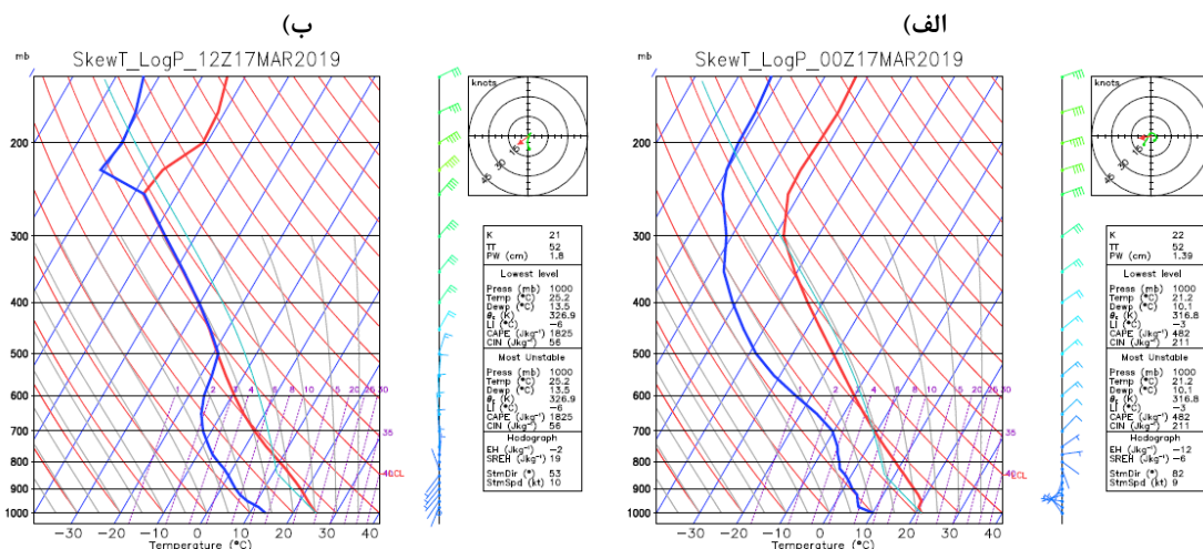
شکل (۷). الف) نمودارهای ترمودینامیکی ساعت ۰۰۰۰ و ب) ۱۲۰۰ گرینویچ روز ۲۶ اسفند ۱۳۹۷ ایستگاه گرگان
