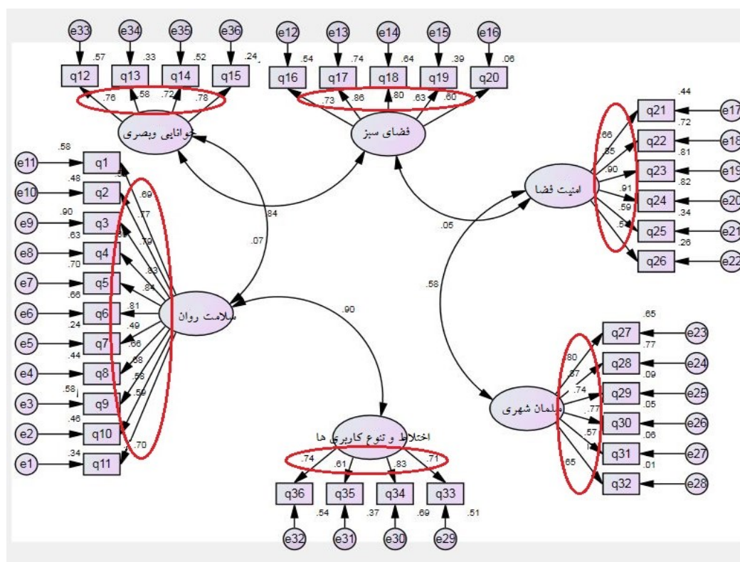
شکل (۲). مدل اندازه‌گیری متغیرهای تحقیق به همراه بار عاملی مربوط به سوالات
