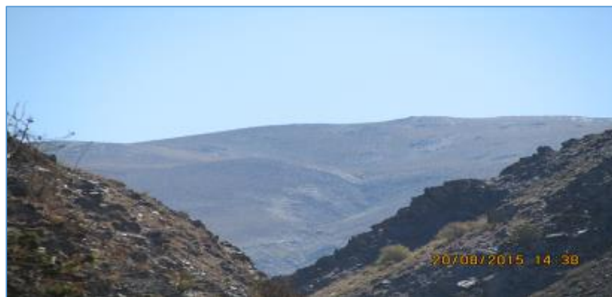
شکل (۹). نمایی از سیرک یخچالی در منطقه مورد مطالعه
