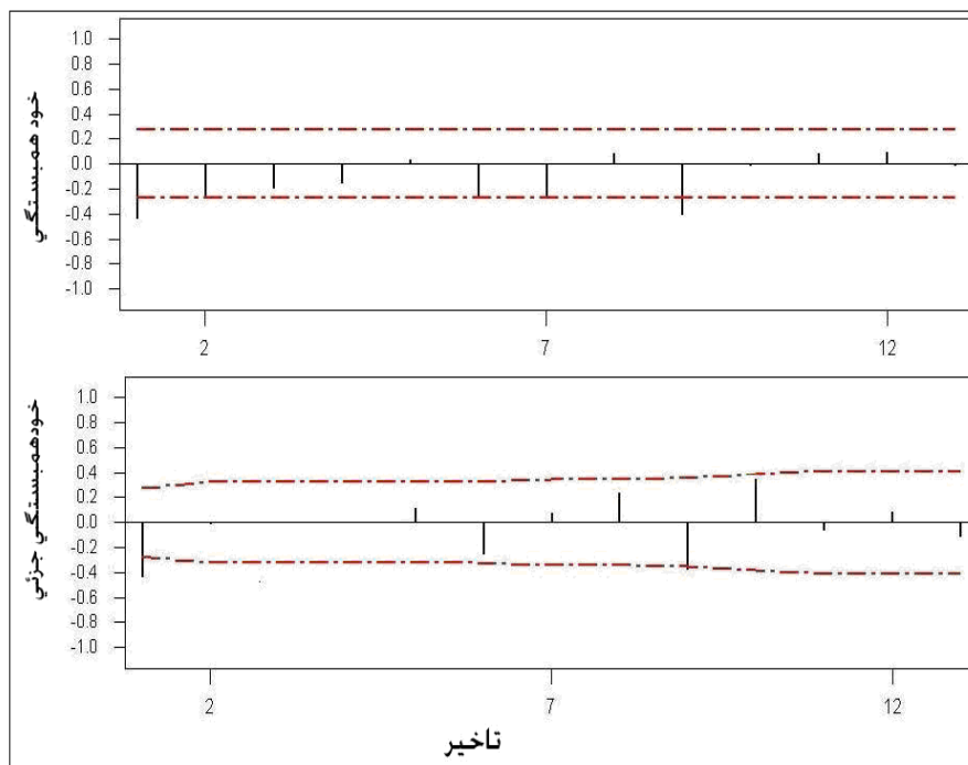
شکل (۳) همبستگی نگار و همبستگی نگار جزئی سری تفاضلی دما (d=۱)
