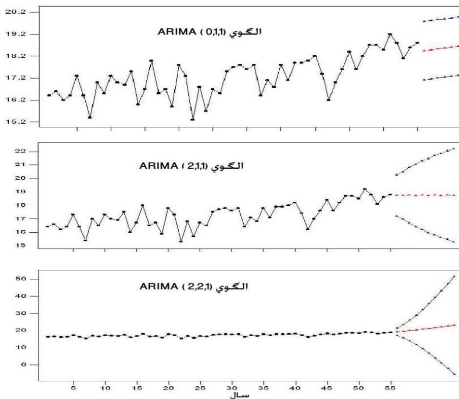
شکل (۴) پیش بینی ۱۰ ساله بر اساس الگوهای (۱ و ۱ و ۰)، (۱ و ۱ و ۲)، (۱ و ۲ و ۲)
