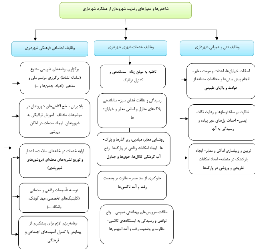
شکل (۳). مدل عملیاتی تحقیق محدوده‌ی مورد مطالعه
