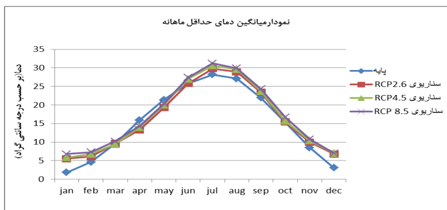
شکل (۲). مقایسه میانگین دمای حداقل در دوره پایه (۱۹۸۴-۲۰۰۵) و دوره آینده (۲۰۲۰-۱۰۳۹) تحت سه سناریوی RCP 2.6، RCP 4.5، و RCP 8.5
