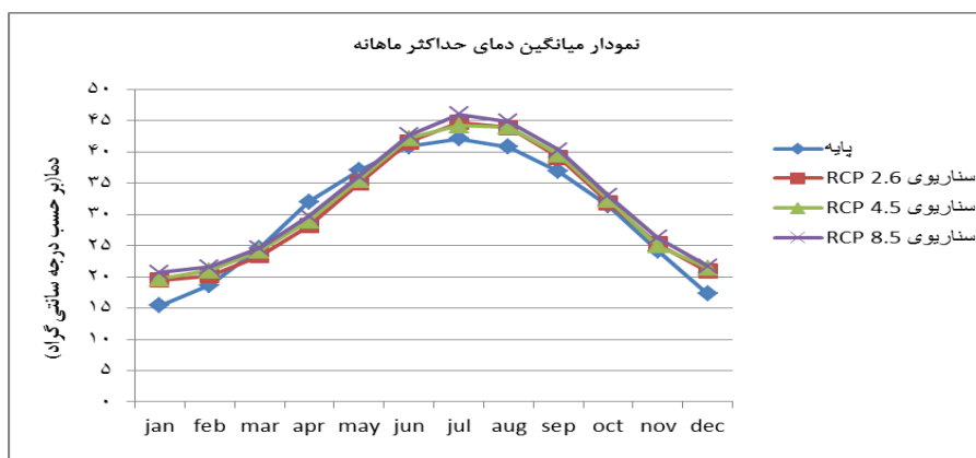
شکل (۳). مقایسه میانگین دمای حداکثر در دوره پایه (۱۹۸۴-۲۰۰۵) و دوره آینده (۲۰۲۰-۱۰۳۹) تحت سه سناریوی RCP 2.6، RCP 4.5، و RCP 8.5.
