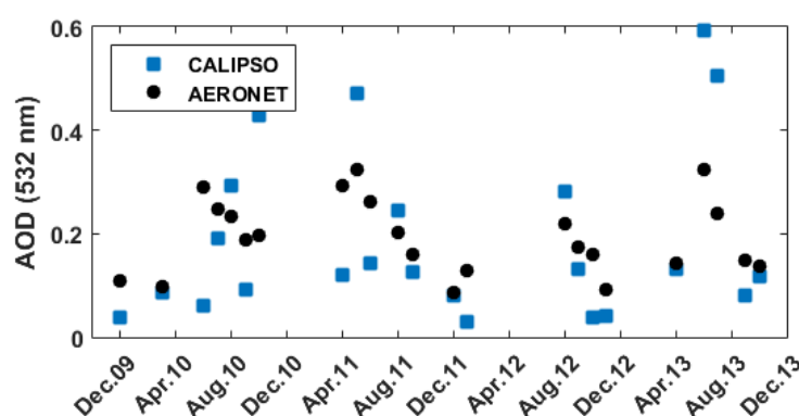
شکل (۶): نمودار سری زمانی میانگین ماهانه عمق اپتیکی هواویز اندازه‌گیری شده توسط سنجنده کالیپو و شیدسنج خورشیدی مستقر در دانشگاه تحصیلات تکمیلی زنجان.
