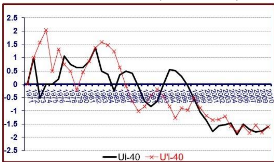
شکل (۳). نمودار تعیین نقاط جهش چهل ساله بارش، به روش من-کندال، ایستگاه ارومیه
