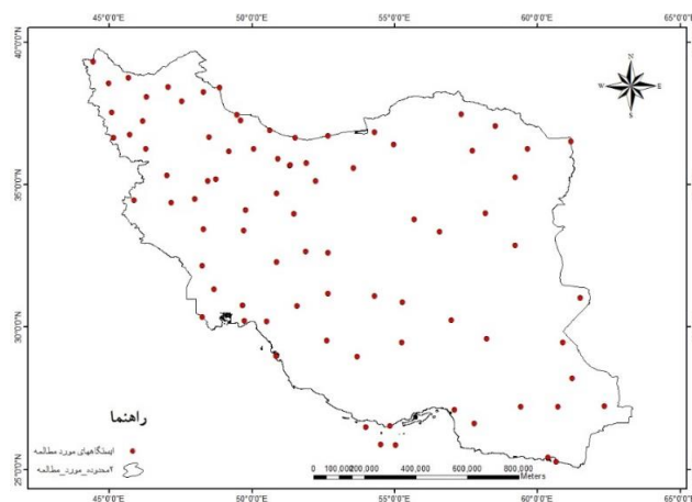
شکل (۱). موقعیت ایستگاه‌های مورد مطالعه
