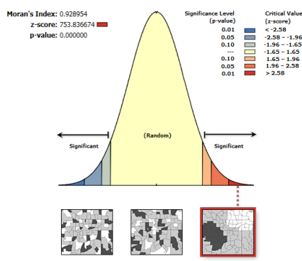
شکل (۸) الگوی خوشه‌ای خشکسالی بسیار شدید
