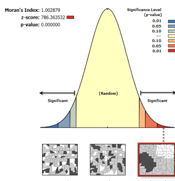
شکل (۴) الف) الگوی خوشه‌ای خشکسالی متوسط
