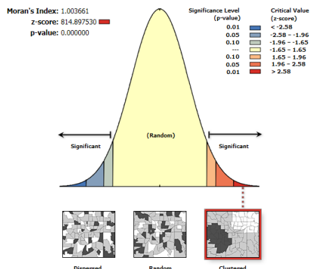
شکل (۶) الگوی خوشه‌های خشکسالی شدید
