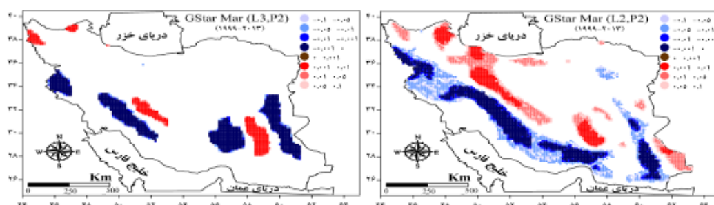
شکل (۳). نقشه‌های خودهمبستگی فضایی VIMFC ژانویه تا مارس بر روی ایران طی دوره اول ۱۹۹۸-۱۹۷۹ (P1) و دوم ۲۰۱۳-۱۹۹۹ (P2). منظور از L1 لایه اول، L2 لایه دوم، L3 لایه سوم است.
