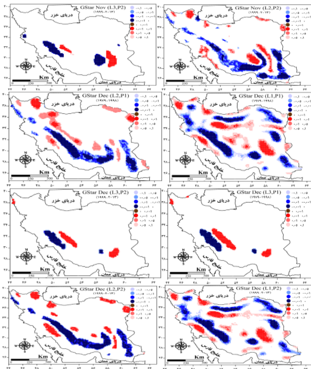
شکل (۶). نقشه های خودهمبستگی فضایی VIMFC ماههای اکتبر تا دسامبر بر روی ایران طی دوره اول ۱۹۷۹-۱۹۹۸ و دوم ۲۰۱۳-۱۹۹۹ (P1) و (P2)
