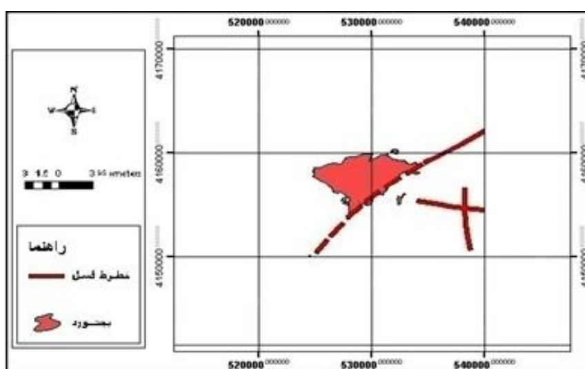
شکل (۵): خطوط گسل بابامان در شهرستان بجنورد
