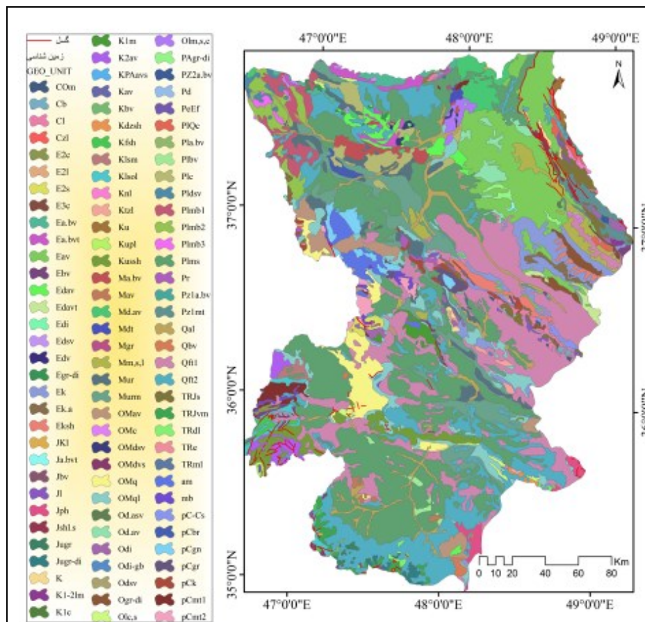
شکل (۳). لایه لیتولوژی حوضه آبریز قزل‌اوزن (سازمان زمین‌شناسی کشور)
