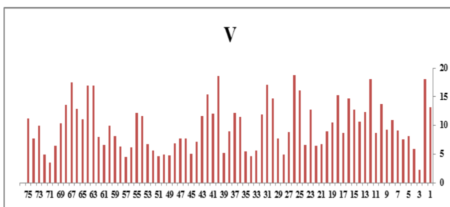
شکل (۹). مقادیر نسبت عرض دره به ارتفاع دره ( V ) برای دره های شناسایی شده در منطقه مورد مطالعه.
