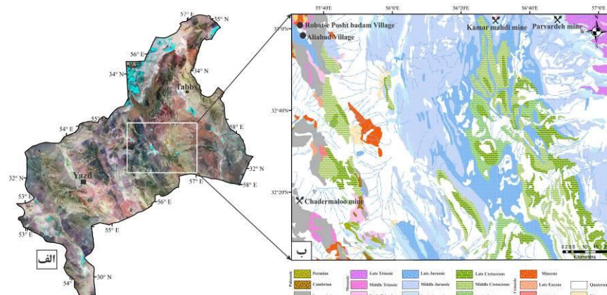
شکل (۱). (الف) موقعیت منطقه مورد مطالعه بر روی تصویر ماهواره ای TM استان یزد و (ب) نقشه زمین شناسی منطقه مورد مطالعه بر گرفته از نقشه ۱/۲۵۰۰۰۰ آبدوخی (آقائباتی و سعیدی، ۱۳۹۰).
