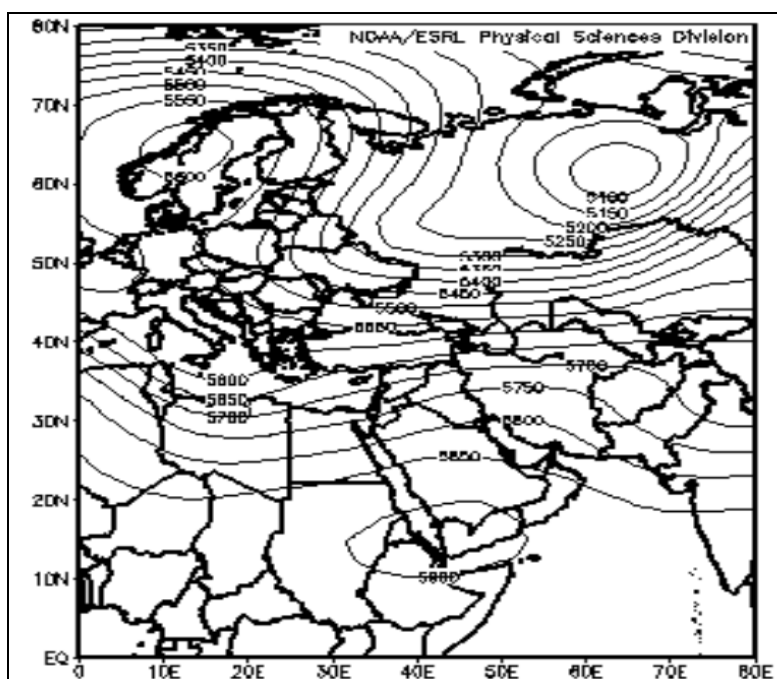
شکل (۷). نقشه الگوی تراز کم عمق (ارتفاع تراز سطح ۵۰۰ هکتوپاسکال)
