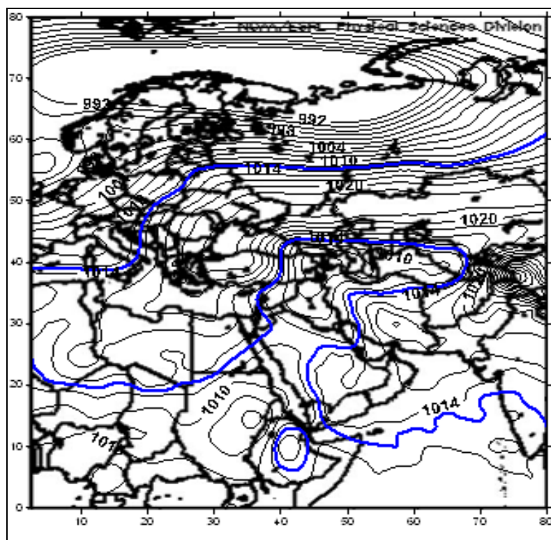
شکل (۵). نقشه الگوی سردچال جو بالایی (فشار سطح دریاهای آزاد)
