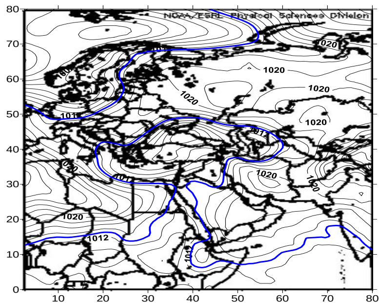
شکل (۶). نقشه الگوی تراف عمیق (الف: سطح ۵۰۰) و (ب: فشار سطح دریاهای آزاد)
