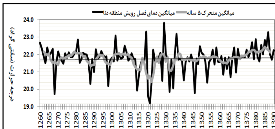
شکل (۷) مقدار میانگین دمای بازسازی شده اردیبهشت - شهر یور، بر اساس گاه شناسی باقیمانده سه رویشگاه سی سخت، میمند و یاسوج جنگل های منطقه دنا در ارتفاعات زاگرس مرکزی ایران، طی یک دوره ی ۱۳۱ ساله (۱۲۶۰-۱۳۹۰)
