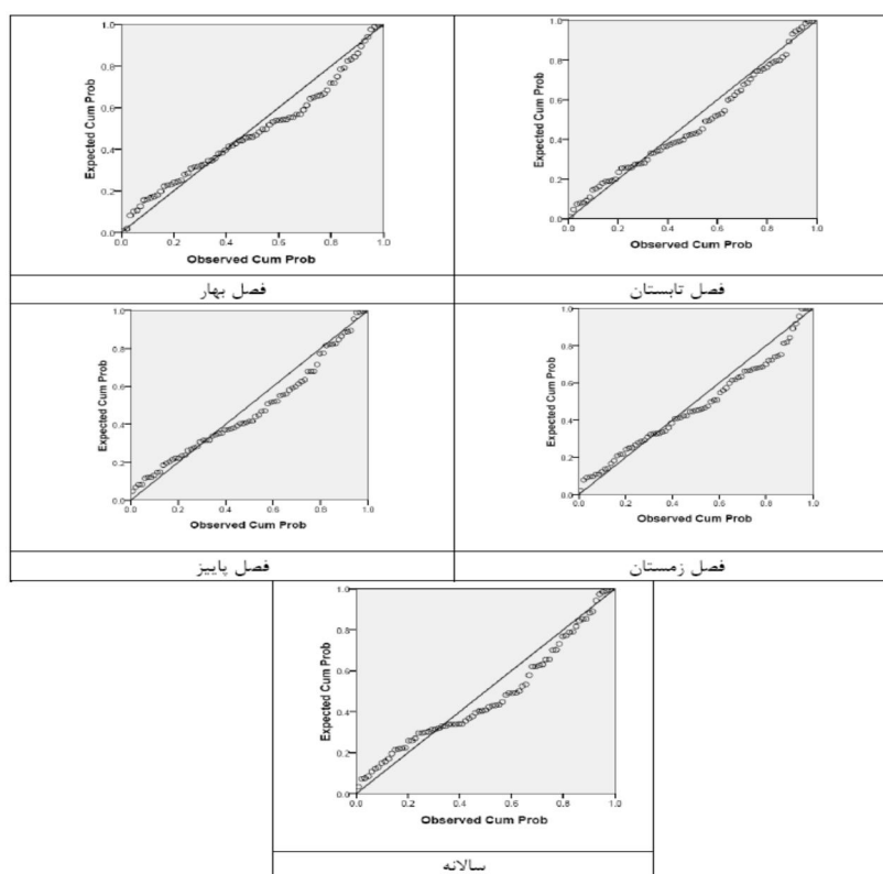
شکل (۲) نمودار P-P Plot جهت آزمون نرمال بودن خطاها در بارش های سالانه و فصلی استان کردستان
