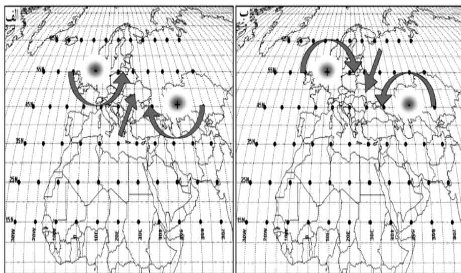
شکل (۲) الگوی دریای شمال-خزر الف: فاز منفی ب: فاز مثبت (کاکاپور به نقل از کوتیل و بناروش، ۱۳۹۰)
