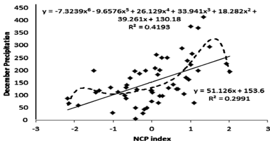
شکل (۴) میزان تأثیرپذیری بارش ایستگاه رشت با الگوی پیوند از دریای شمال-خزر در ماه دسامبر
