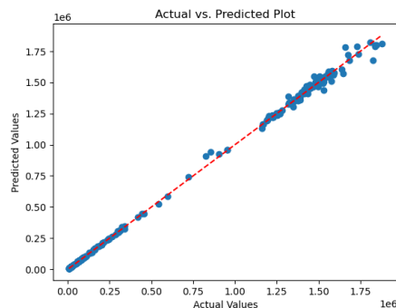
شکل ۸. نمودار پراکندگی XGB
