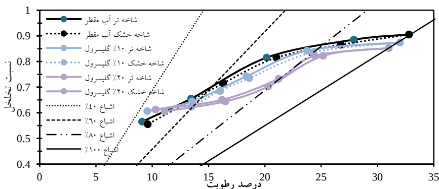
شکل ۶. تغییرات نهایی نسبت تخلخل با درصد رطوبت (مسیرهای تورمی و انقباضی) طی چرخه‌های متوالی تر و خشک شدن آب مقطر و محلول‌های ۱۰ و ۲۰ درصد گلیرول
