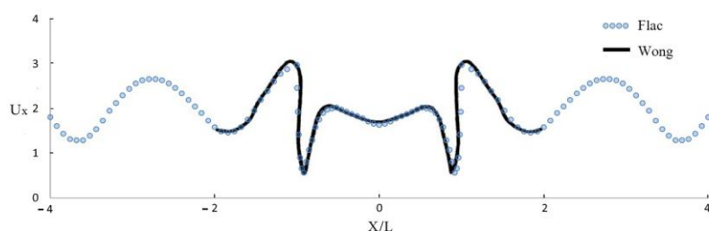
شکل ۱. صحت‌سنجی نتایج تحلیلی نرم‌افزار FLAC برای توپوگرافی دره ( R=25 , \lambda/R=2 ) موج قائم (SV)
