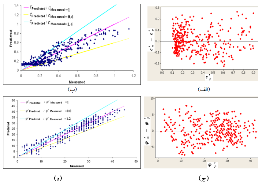
شکل ۷. نمودار ارزیابی میزان خطای برآورد برای خاک‌های منطقه جنوب تهران در حالت زهکشی شده (بر اساس روابط ۱۲ و ۱۳) الف) مقادیر چسبندگی برآورد شده و میزان خطای باقی‌مانده مرتبط با هر برآورد ب) نسبت مقادیر چسبندگی برآورد شده به مقادیر چسبندگی اندازه‌گیری شده شده ج) مقادیر زاویه اصطکاک داخلی برآورد شده و میزان خطای باقی‌مانده مرتبط با هر برآورد د) نسبت مقادیر زاویه اصطکاک داخلی برآورد شده به مقادیر زاویه اصطکاک داخلی اندازه‌گیری شده
