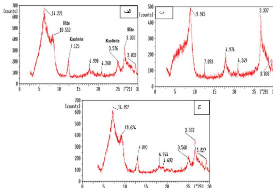
شکل ۳. طیف انکسار اشعه X در نمونه A 18 را در سه حالت الف) نمونه خشک شده در دمای طبیعی، ب) نمونه حرارت داده شده ج) نمونه عمل آوری شده با اتیلن گلیکول نشان می‌دهد، چنان‌که ذکر شد کانی‌های رسی موجود در سنگ‌های مارنی ساختگاه سد از نوع ایلیت و کائولینیت هستند.
