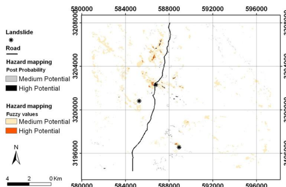
شکل ۱۳. مناطق دارای پتانسیل لغزش، حاصل از هر دو روش فازی و هیبرید؛ چنان که مشاهده می شود مناطق با پتانسیل زیاد لغزش در هر دو روش با هم منطبق هستند
