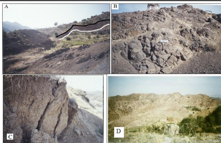
شکل ۲. A) یک زمین لغزش در منطقه را نشان می‌دهد که تاج لغزش با خط مشکی و قله زمین لغزش با خط سفید نشان داده شده است B) هوازدگی پوست‌پیزی که در منطقه مشاهده می‌شود و در سنگ‌های آگلومرا در بالا نشان داده شده است C) ترک‌های ناشی از لغزش در منطقه بررسی شده D) سنگ‌های آلتزه شده در منطقه
