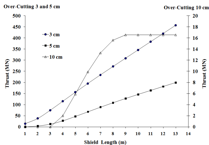
شکل ۳. تغییرات تراست لازم برای غلبه بر اصطکاک بدنه در مقابل طول سپر برای شرایط ژئومکانیکی کمینه در کیلومتر ۳۱۶۰۰-۳۱۶۰۳ و ۳۴۹۰۰-۳۴۹۰۳
