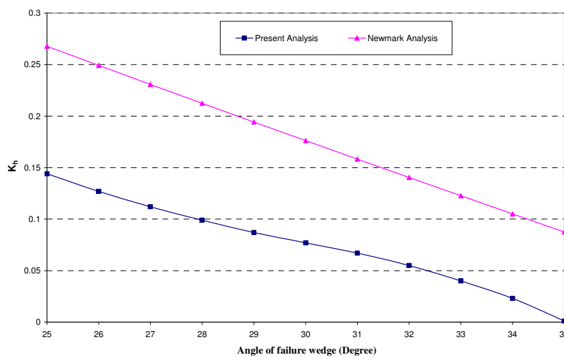
شکل ۹. تغییرات ضریب شتاب لرزه‌ای افقی تسلیم در برابر زاویه گوه گسیختگی
