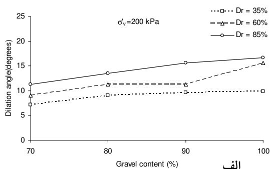
شکل ۲۰. تغییرات زاویه اتساع در مقابل مقدار شن در تراکم‌های نسبی مختلف برای سربارهای (الف) ۱۰۰ کیلوپاسکال
