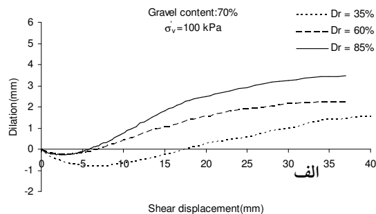
شکل ۵. نمودار الف) تنش برشی در مقابل جابه‌جایی افقی،
