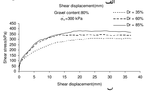
شکل ۱۰. ب) جاب‌جایی قائم در مقابل جاب‌جایی افقی
