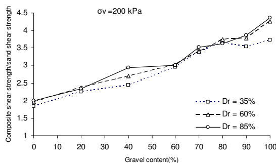
شکل ۱۸. تأثیر تراکم نسبی بر نسبت
