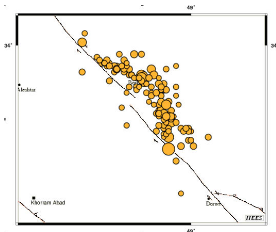
شکل ۶. توزیع مکانی پس لرزه‌های دوماه زمین‌لرزه ۱۳۸۵/۱/۱۱ درب آستانه سیلاخور
