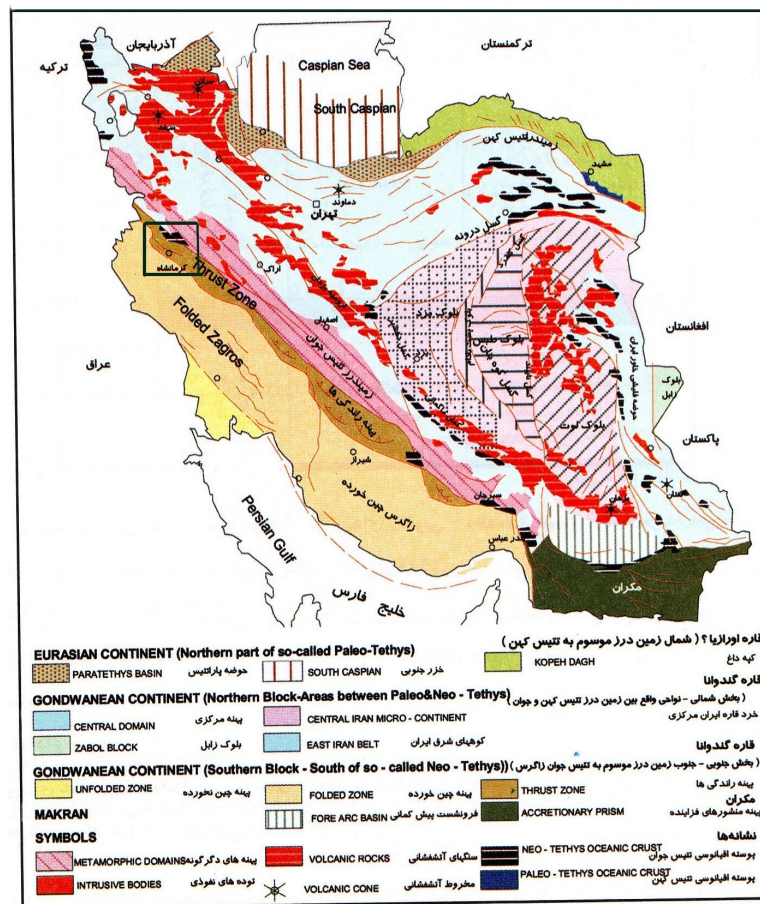
شکل ۲. پهنه‌های رسوبی - ساختار عمده ایران [۲۱]
