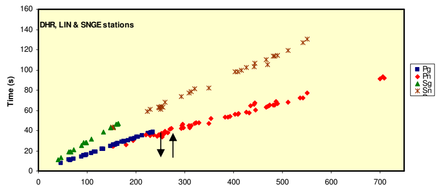
شکل ۱۵. نمودار زمان-مسافت موج‌های P و S به‌روش دو ایستگاهی در امتداد مسیرهای دهرش، لاین و سندج شکل ۱
