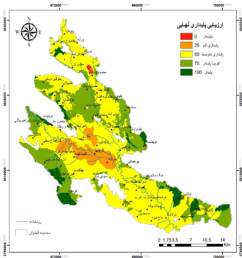
شکل ۳. نقشه پایداری نهایی آبخیز کرمانشاه بر اساس روش تحلیل سلسله مراتبی Fig. 3. Final sustainability map of Kermanshah Aquifer based on the AHP
