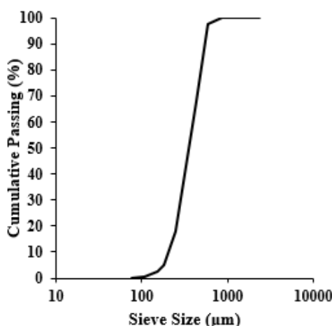
شکل ۱. منحنی دانه‌بندی ماسه مورد استفاده مطابق با استاندارد ASTM C136-06.
