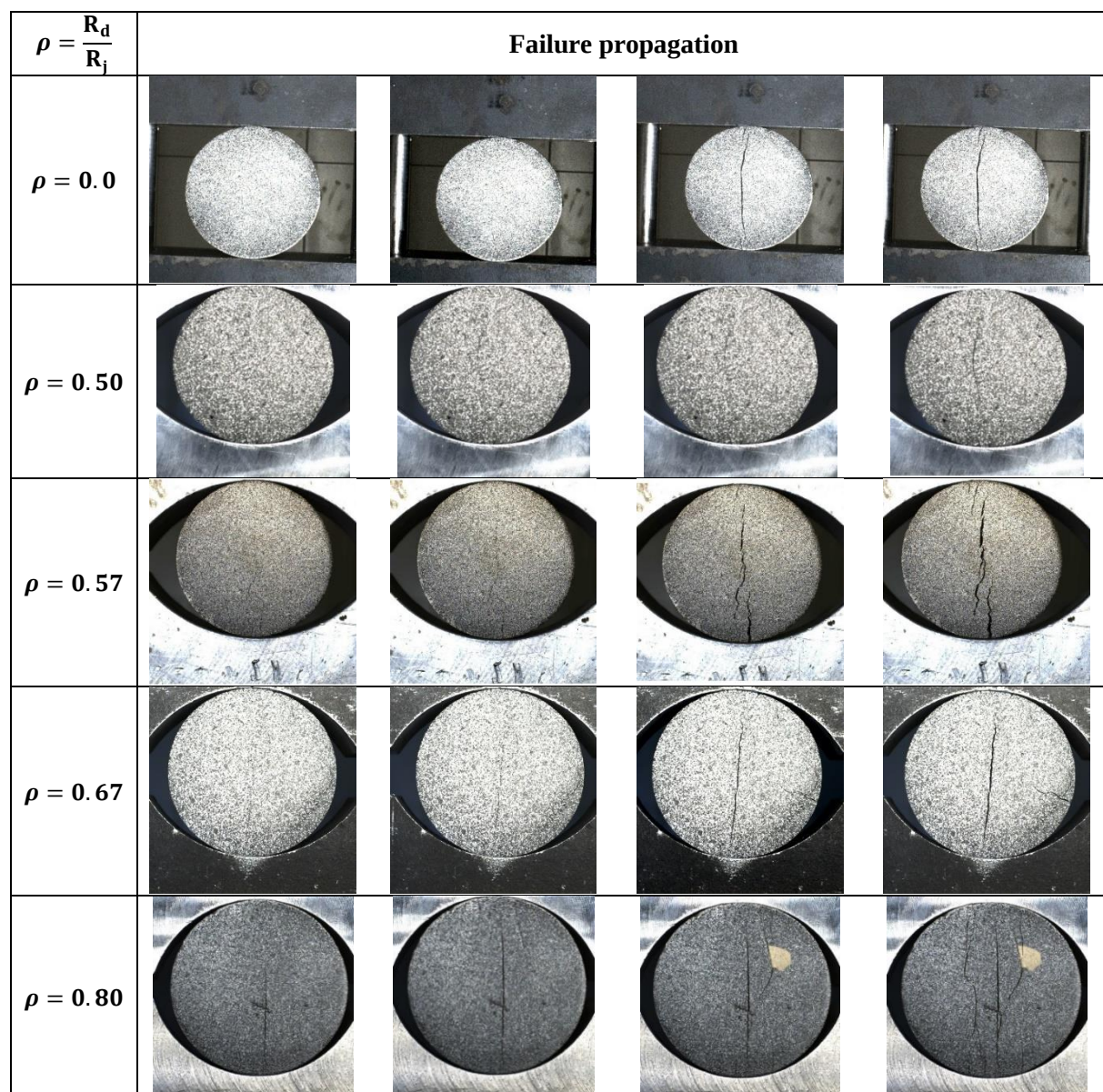
شکل ۴. ثبت مراحل گسترش ترک در نمونه دیسک‌های برزیلی در فک‌های بارگذاری با نسبت انحنا متفاوت.
