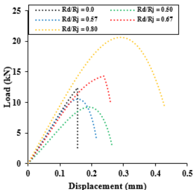
شکل ۵. تأثیر تغییر نسبت انحناء صفحات بارگذاری بر نتایج نمودار نیرو - جابه جایی Fig. 5. Effect of the variation in the ratio of specimen radius to jaw radius ( \rho ) on the Load-displacement response
