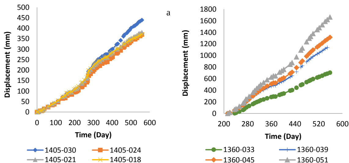
شکل ۱. گراف جابه‌جایی ثبت شده برای دیواره معدن در مقابل روز مطابق با مدل ماکسول، a. تراز ۱۴۰۵ و b. تراز ۱۳۶۰، تاریخ شروع قرائت: ۹۷/۸/۸
