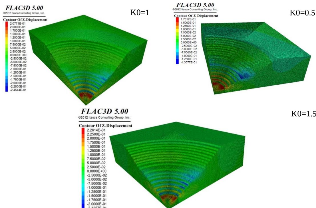
شکل ۸. کنتور جابه‌جایی‌ها در راستای Z در سناریوی سوم برای نسبت‌های تنش افقی به قائم ۱/۵ و ۱، ۰/۵ و ۱.۵ Fig. 8. Displacement contours in the Z direction in Scenario 3 for horizontal-to-vertical stress ratios of 0.5, 1, and 1.5
