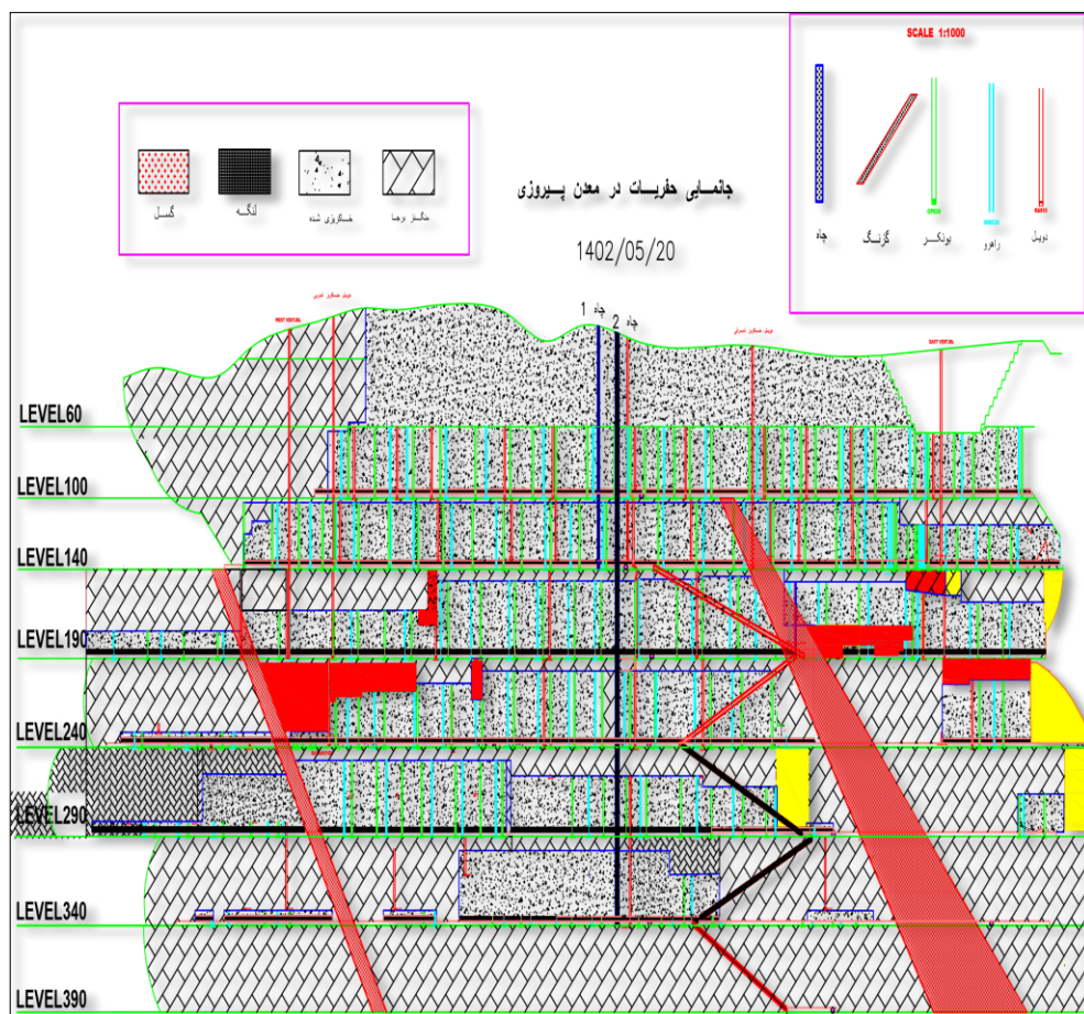
شکل ۱. پروفیل طولی از بلوک پیروزی به همراه کانسار منگنز، عوارض زمین‌شناسی و حفیات انجام شده
